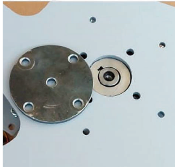
Centrado de disco
