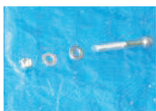
TORNILLO M8x60 TCEI ZN ROSETA 8.4x16 H1.6 ZN TUERCA AUTOBL. M8 ZN
